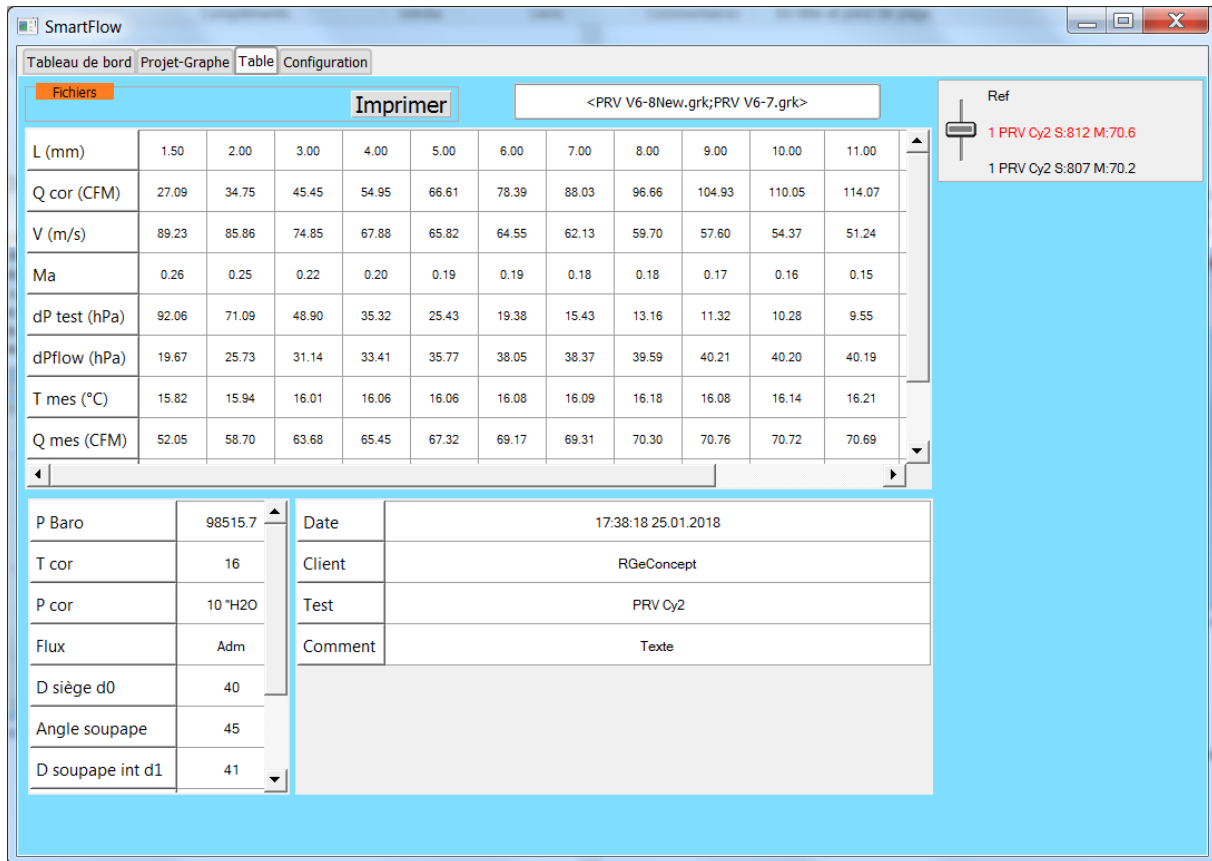
Figure 24 Lecture d'une table d'un projet à 2 courbes. Sélection/visualisation de la 1ere.
