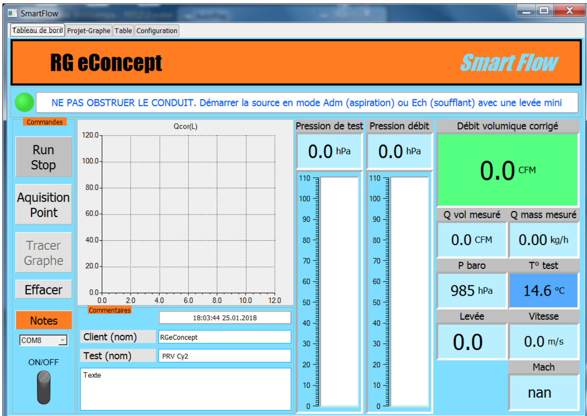
Figure 13 Démarrage et connexion au FCU.
