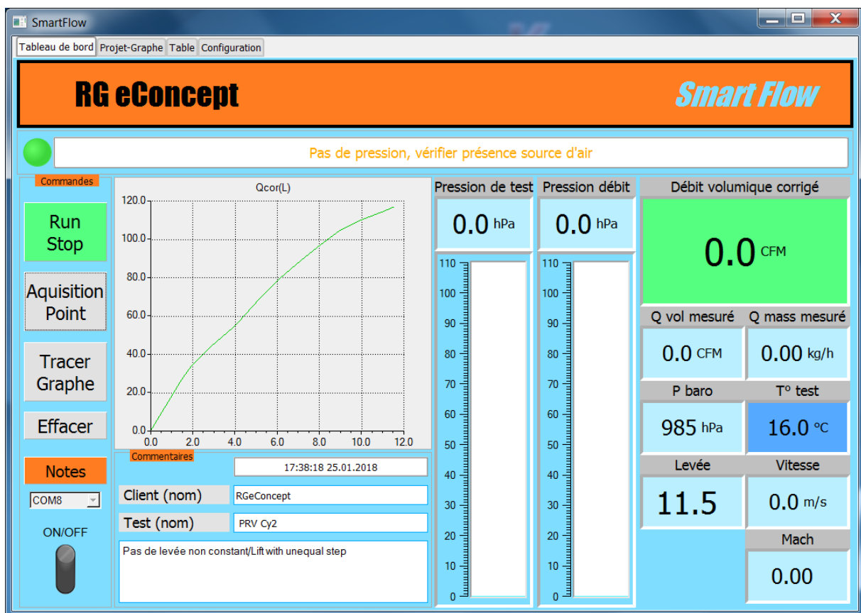
Figure 16 Fin d'acquisition : levée max atteinte et graphe temps réel complet.
