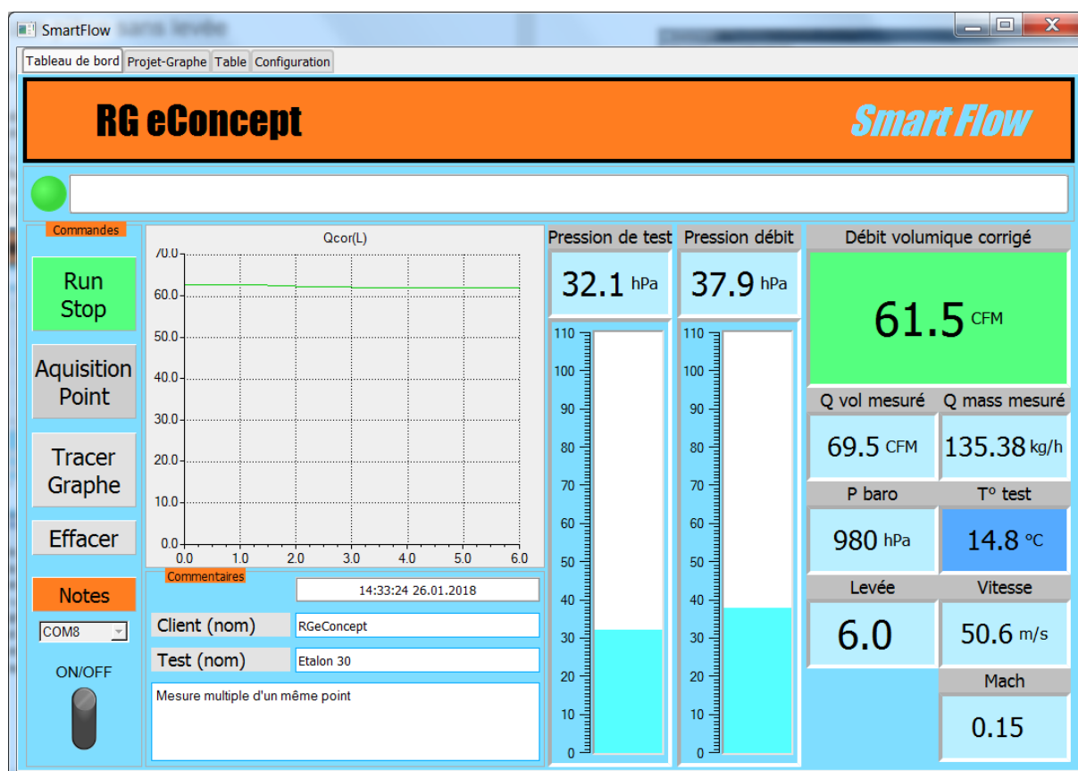
Figure 21 Affichage temps réel d'une pièce sans levée.
