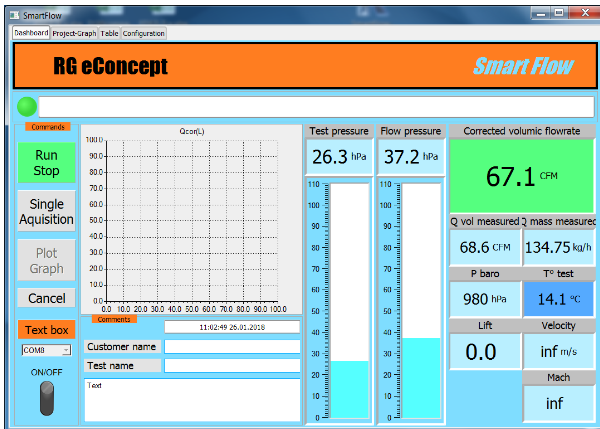
Figure 15 Affichage des paramètres de mesures en temps réel.
