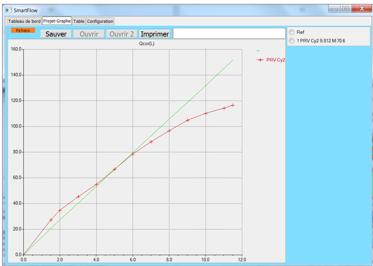
Figure 17 Graphe de la courbe obtenue et courbe de référence. Ecran avant sauvegarde.
